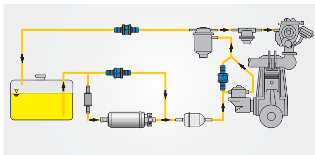
Exemple d'application : Moteur à carburateur avec pompe supplémentaire électrique connectable
